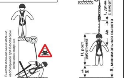
Рис. 11. Расчет высоты свободного пространства под пользователем для безопасной остановки падения
