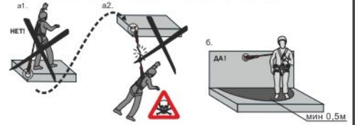
Рис. 9. Использование совместно с амортизаторами
